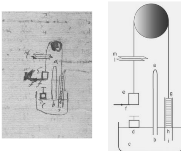
Abb. 13: Kombination von Vakuumexperimenten
