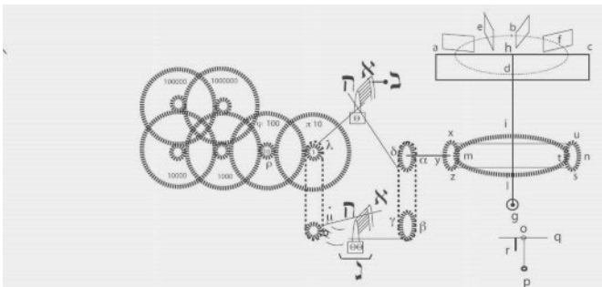
Abb. 4: Skizze des Horologium ventaneum perpetuum
